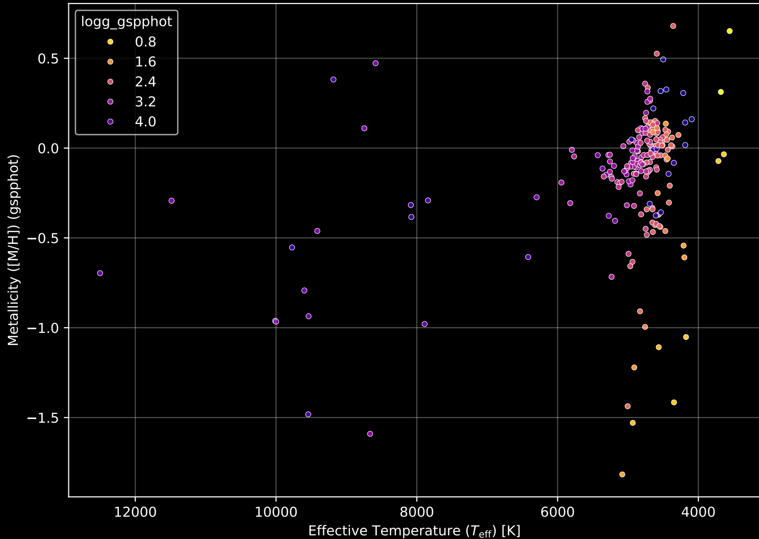
APOGEE DR17 Field: [049+12] Stellar Population Parameters (n= 217)
